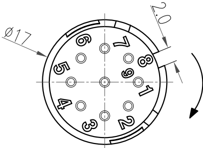
触点排列: 配合面 Contact arrangement: mating side
